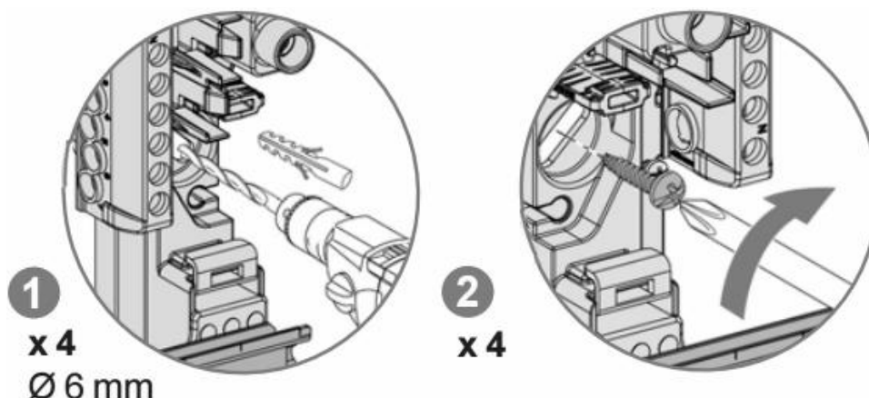
Figure 2. Montage de l'UPG sur un mur
