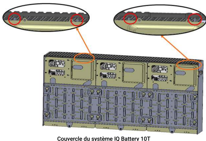
Couvercle du système IQ Battery 10T
