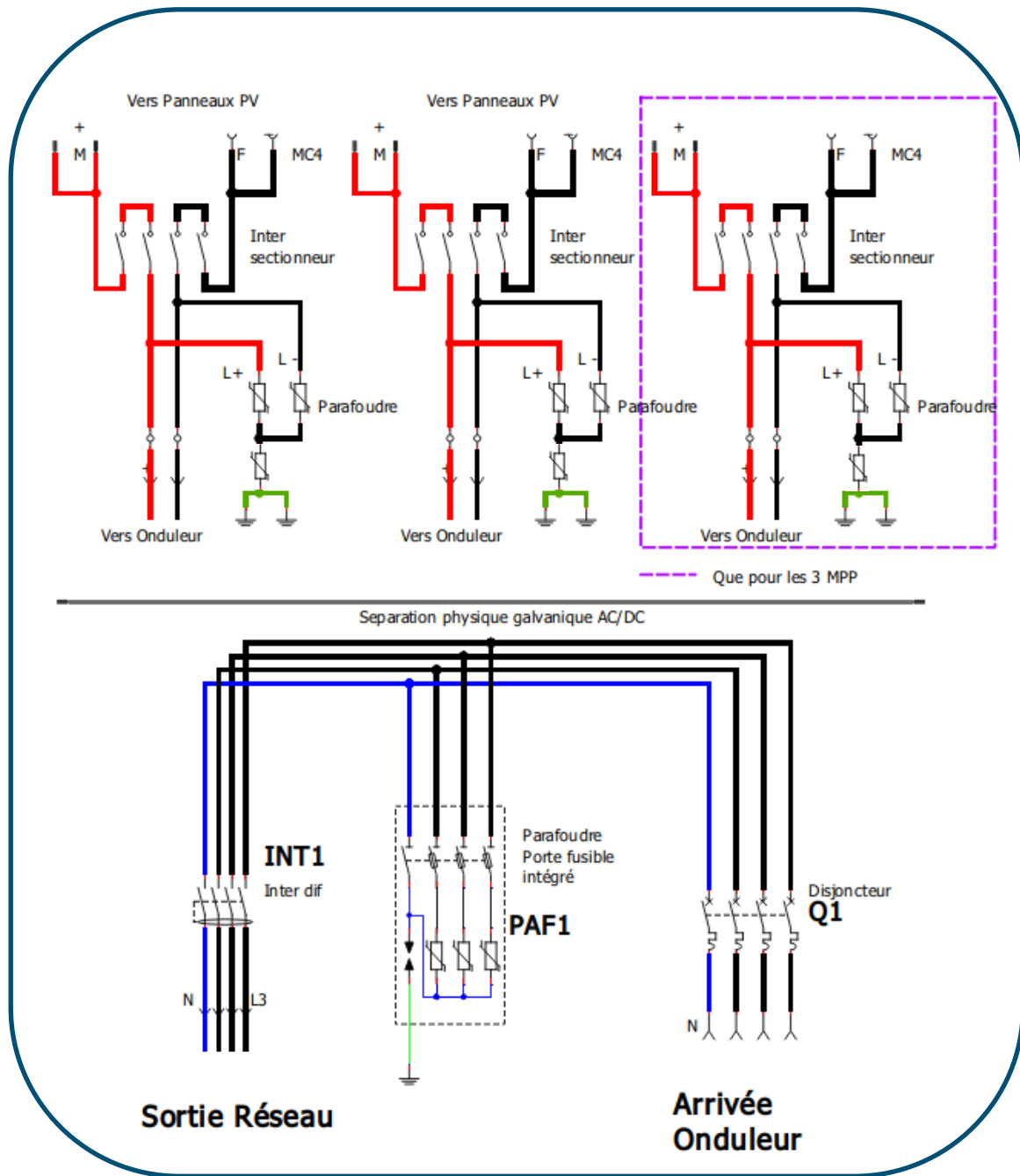
Figure 47 : Schéma de principe coffret AC+DC TRI 1 onduleur 2 MPP (variante à 3 MPP) à 2 strings
