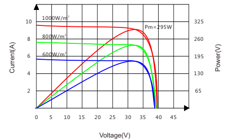
Current-Voltage&Power-Voltage Curve(295W)
