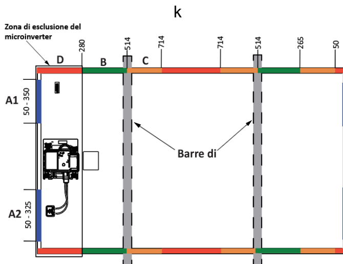
Fig. 1: con supporto della barra di guida
