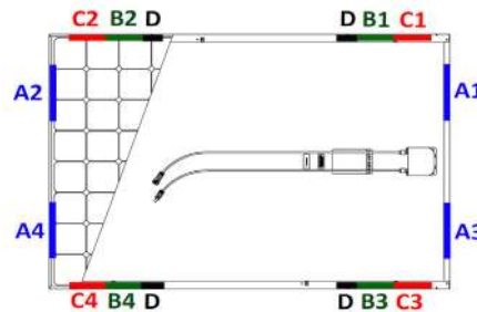
Figure 2 : Position des brides ou attaches de fixation pour les panneaux Maxeon
