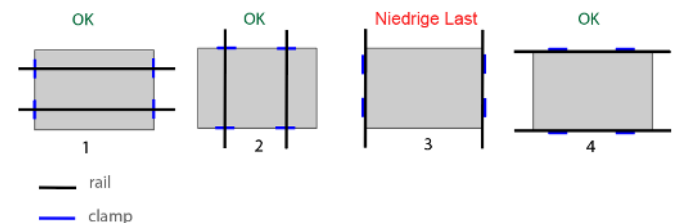
Abbildung 3: Montagekonfigurationen
