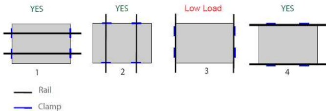
図 3. 架台の構成
